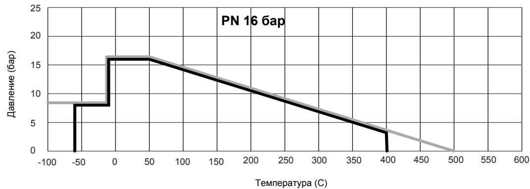
Диаграмма зависимости Давление-Температура
